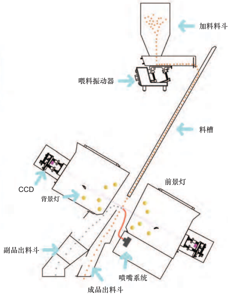
耐用的喷嘴系统
