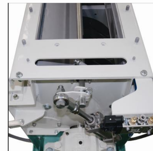
侧向顶置进风口
