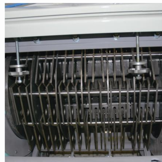
锤片
