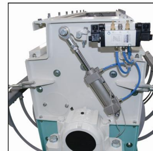
远程控制翻板进料门
